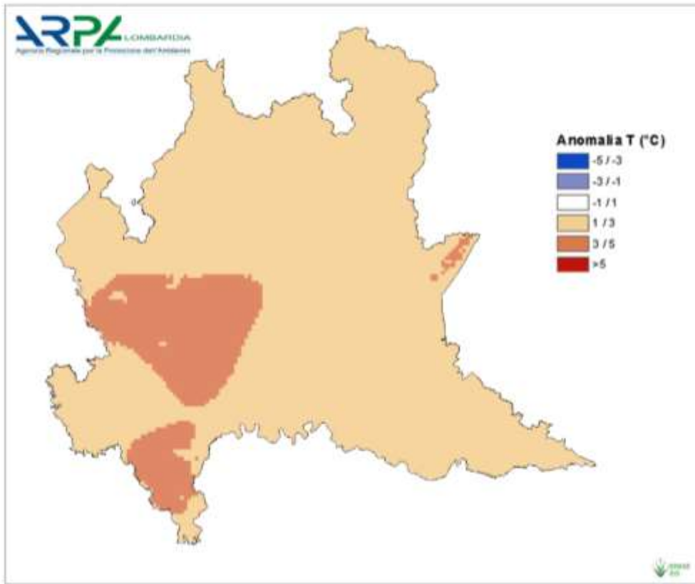
ANOMALIA TEMPERATURA MEDIA DELL'ARIA – GIUGNO 2022
